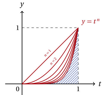
Représentation de la suite (t \mapsto t^n)
